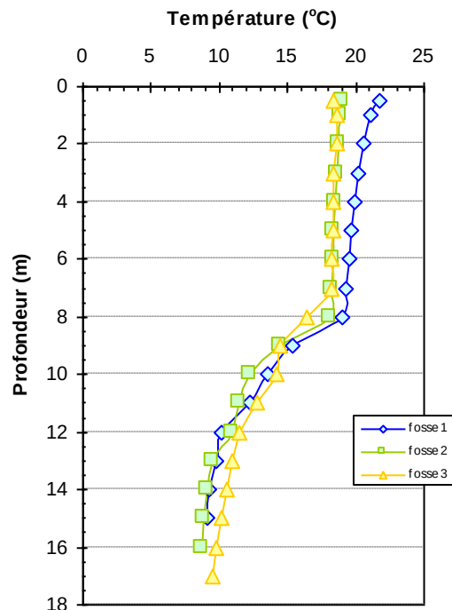
Fig. 7 Profil de température du lac Sept-îles 5 sept. 2007
