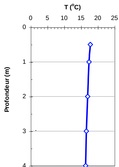
Fig. 9 Profil de temp. lac des Aulnaies 5 sept. 2007
