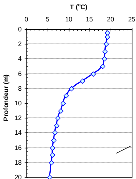
Fig. 8 Profil de température du lac Aux Chiens 5 sept. 2007
